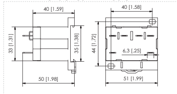
Dimensiones RPA faston-DIN
